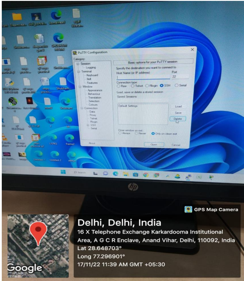
Linux
